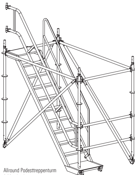
Allround Podesttreppenturm 4,00 m hoch
